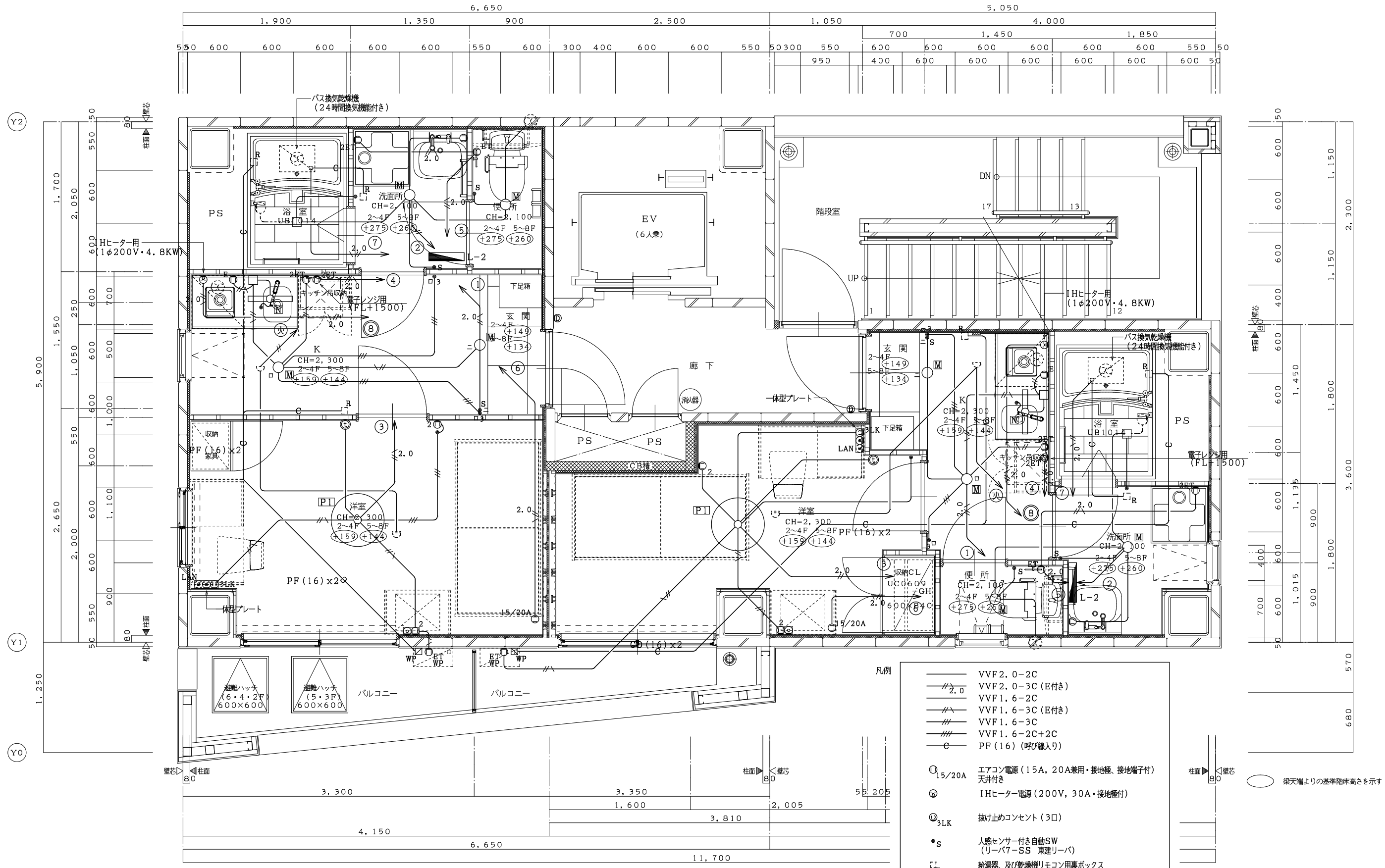
2~6階平面詳細図 S=1:30
